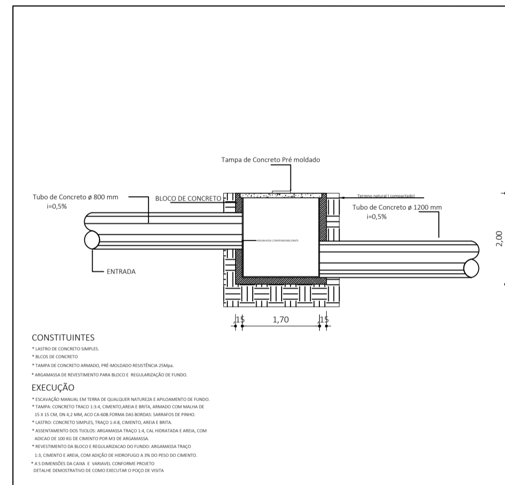
Corte EE' - Poço de Visita 05
