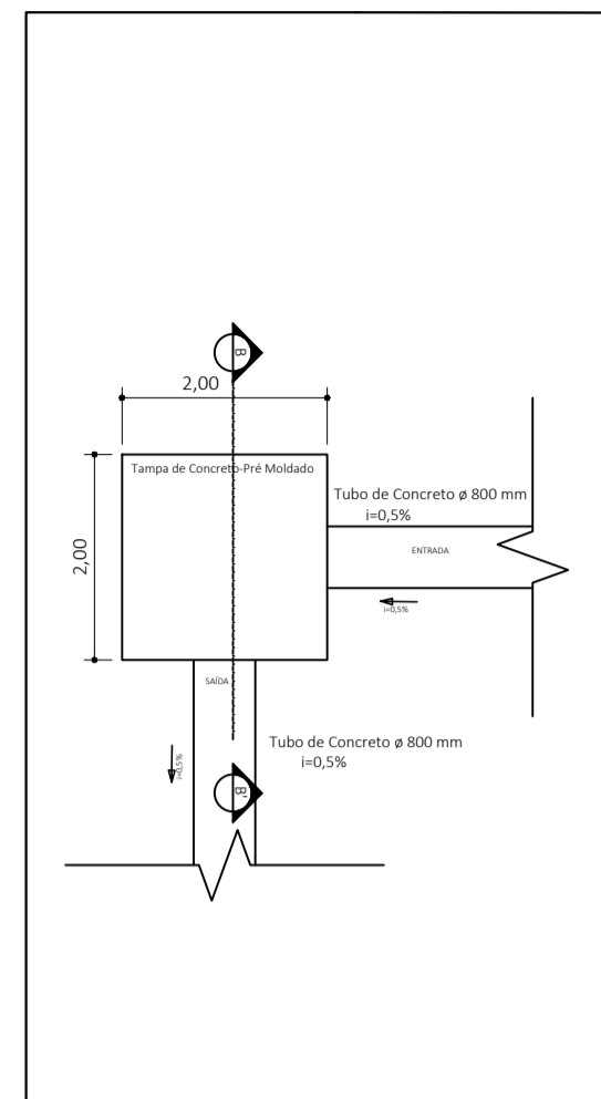
Planta Baixa - Poço de Visita 05
