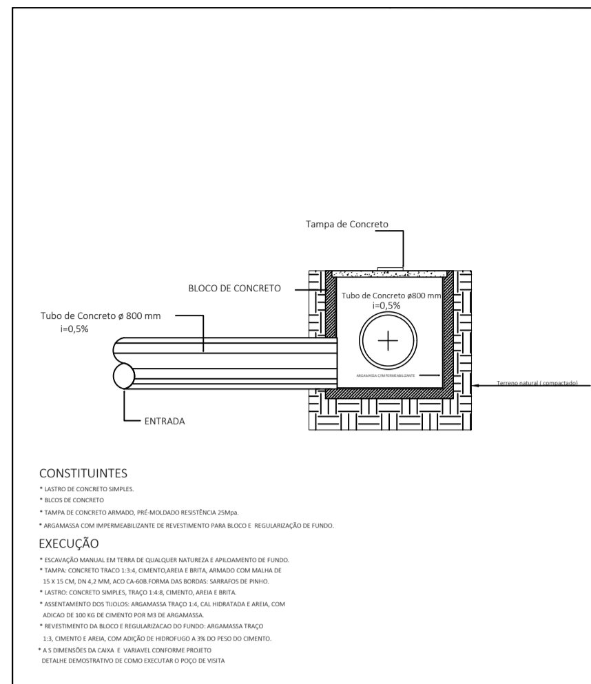
Corte -AA'- Poço de Visita 01
