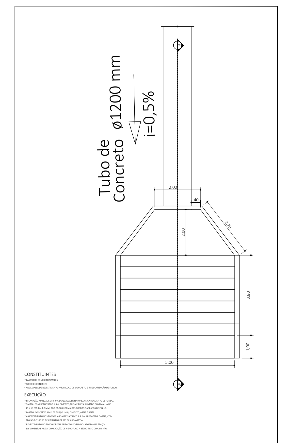
Planta Baixa Dissipador D01
