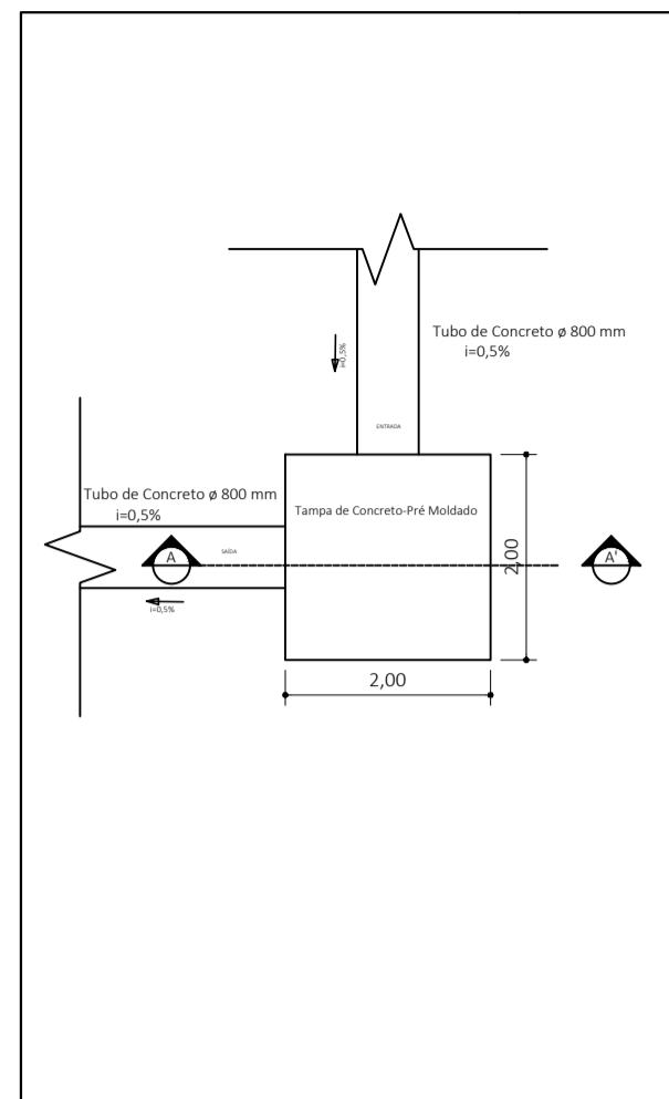
Planta Baixa - Poço de Visita 04
