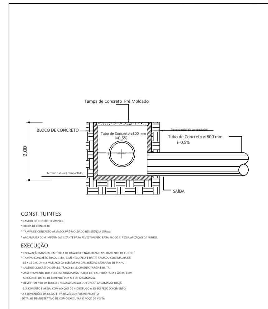
Corte EE' - Poço de Visita 05
