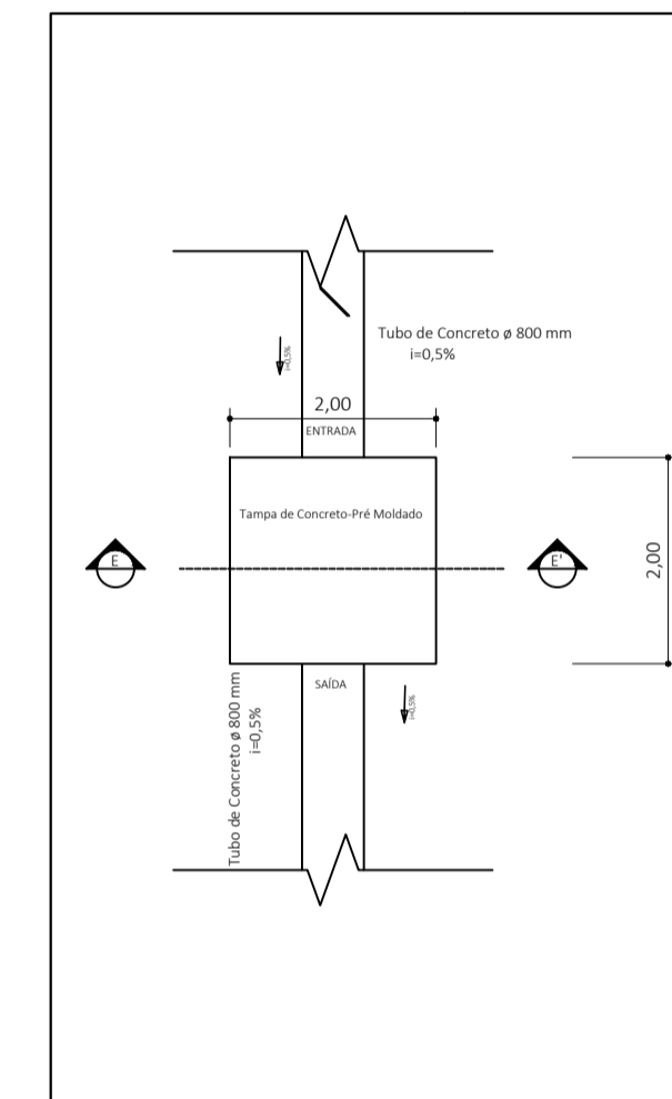
Planta Baixa - Poço de Visita 05
