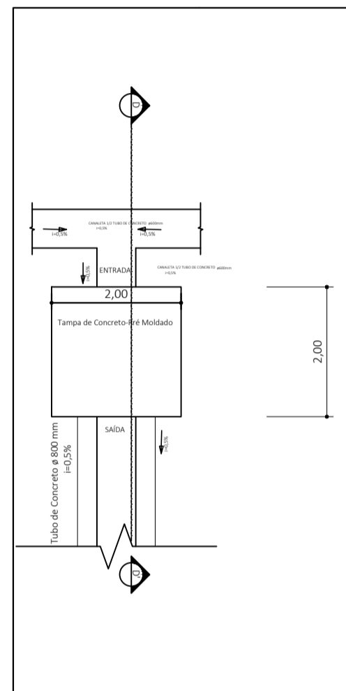
Planta Baixa - Poço de Visita 04
