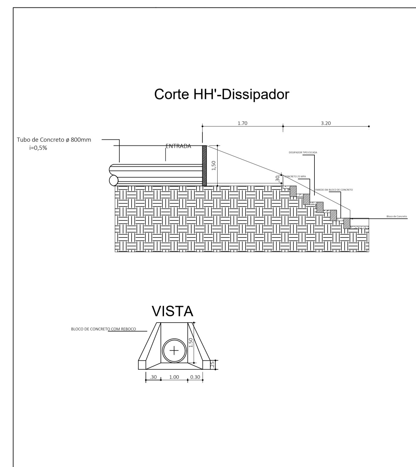
Corte e Vista Dissipador D02
