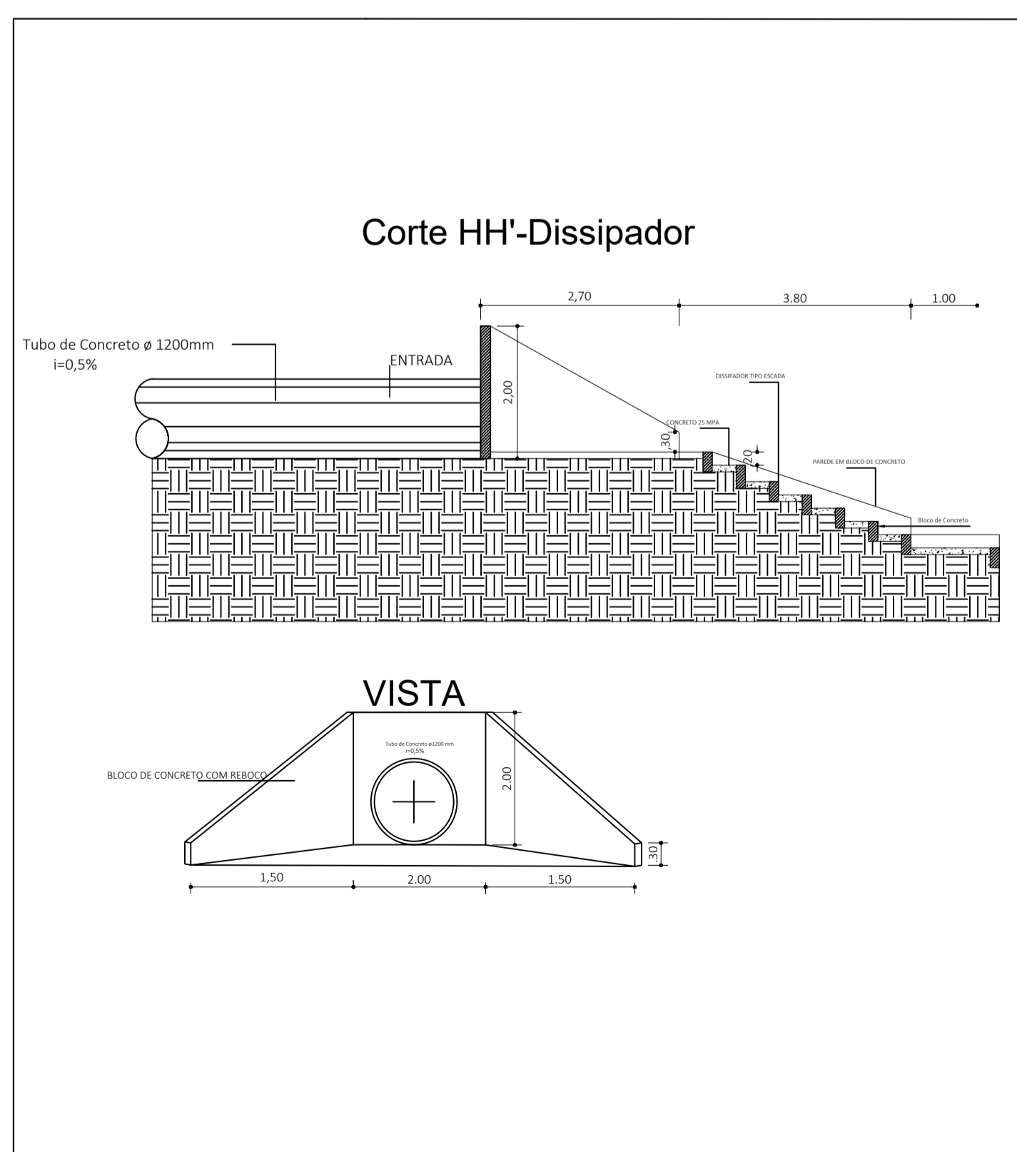
Corte e Vista Dissipador D01
