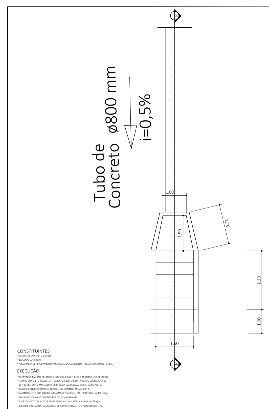
Planta Baixa Dissipador D02
