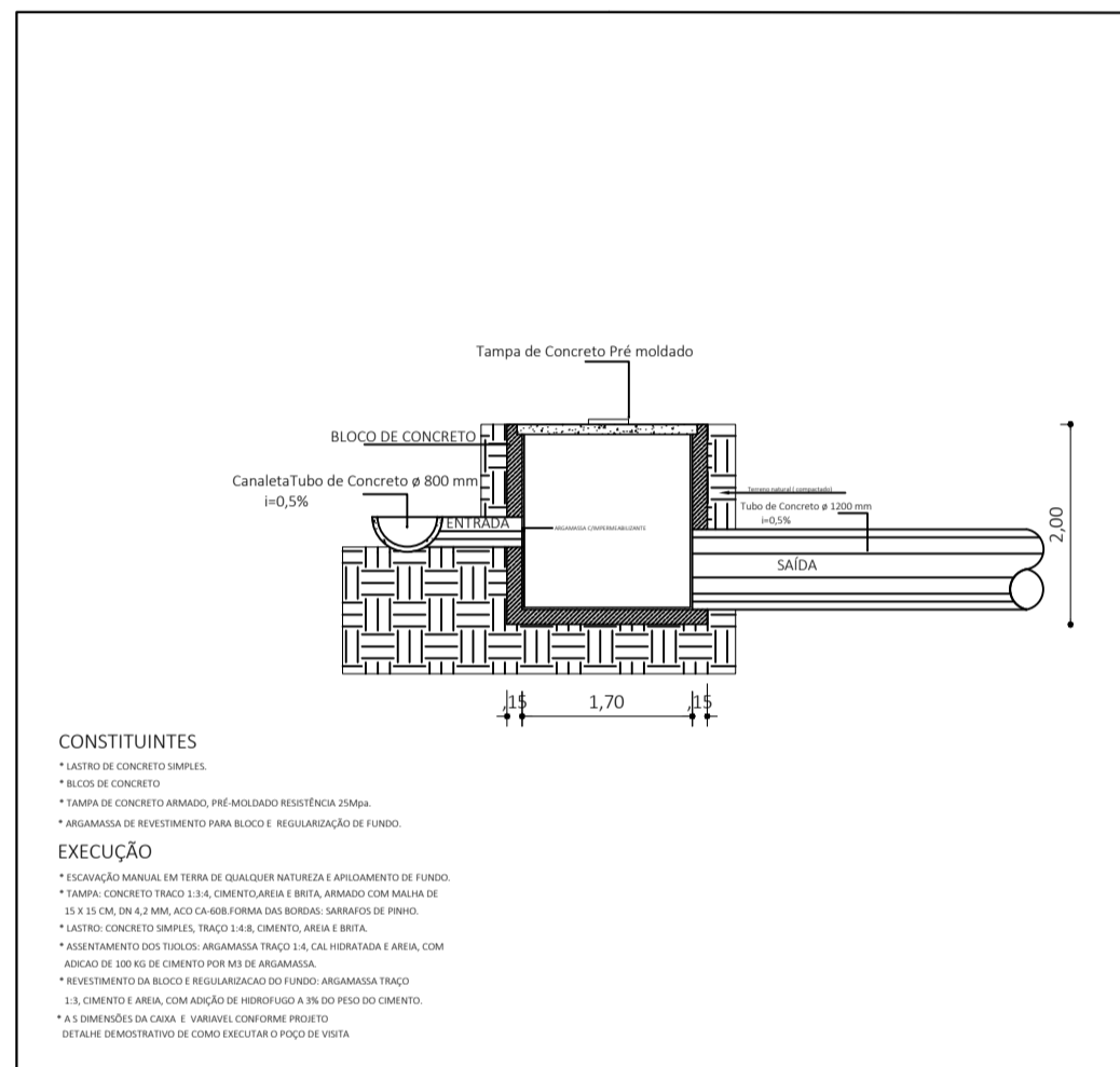
Corte DD' - Poço de Visita 04
