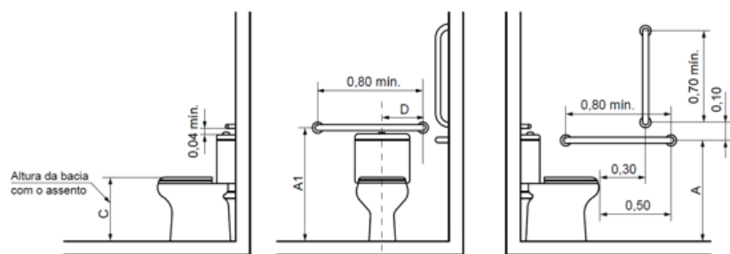
Figura 8 - ilustração retirada da NBR 9050 2015.
