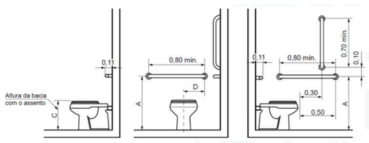
Figura 7 - ilustração retirada da NBR 9050 2015
