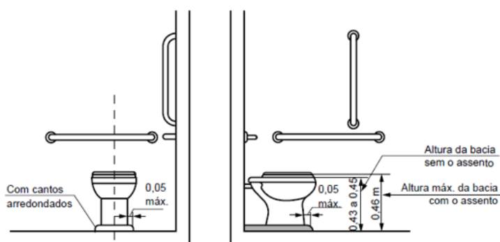
Figura 6 - ilustração retirada da NBR 9050 2015.
